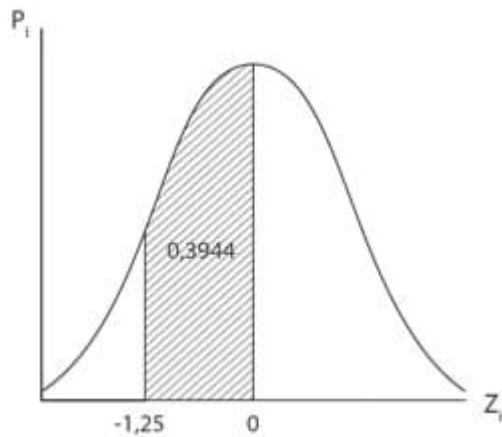
Şekil: Ortalama ile ortalamadan küçük bir değeri arasındaki olasılığın belirlenmesi
