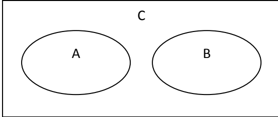
Şekil 1: Birbirini Engelleyen Olaylar.
